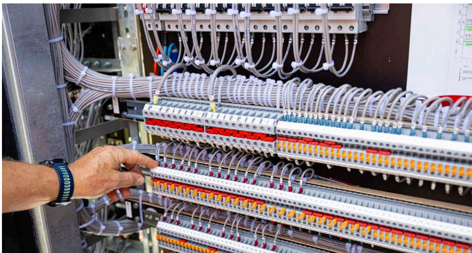
Aanraakveilige relaiskast.
